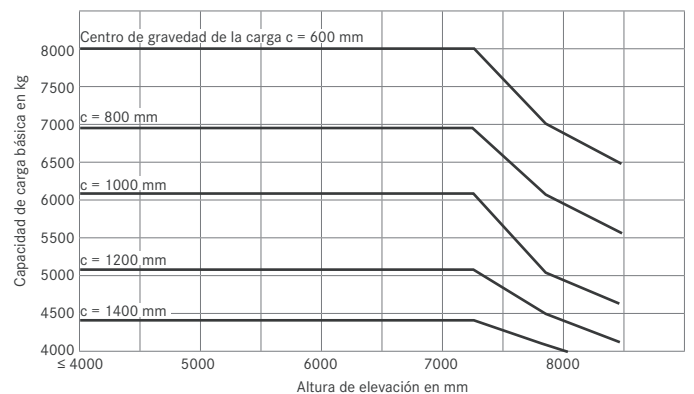
RX 60-80 Mástil Triple
