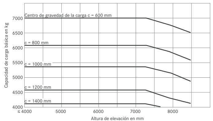
RX 60-70 Mástil Triple
