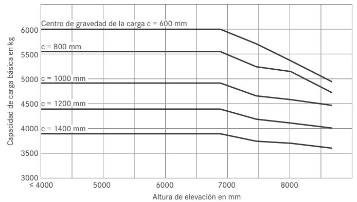
RX 60-60 Mástil Triple
