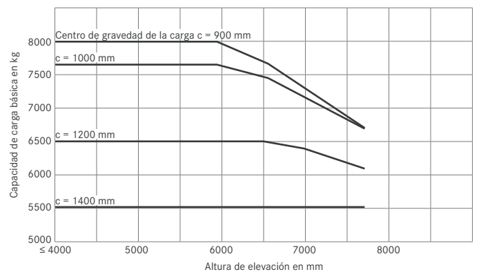
RX 60-80/900 Mástil Triple
