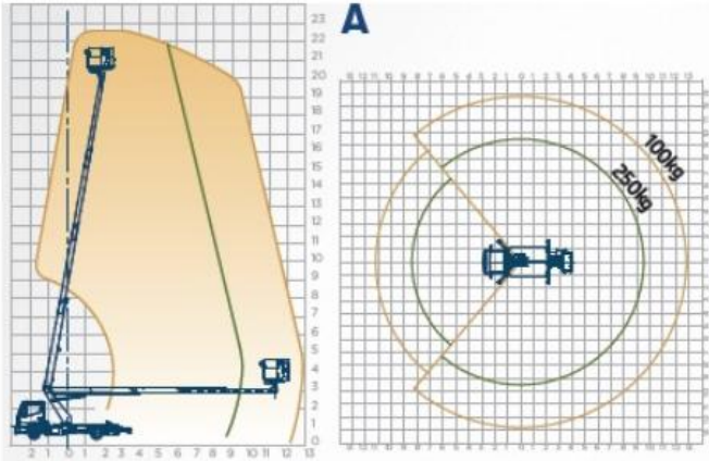
Stabilizzatori chiusi - Closed outriggers
